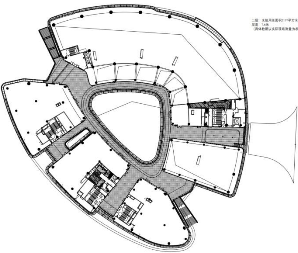
二层平面图
